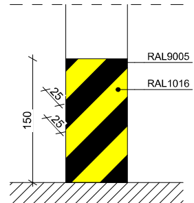
DETAL MALOWANIA SŁUPÓW
